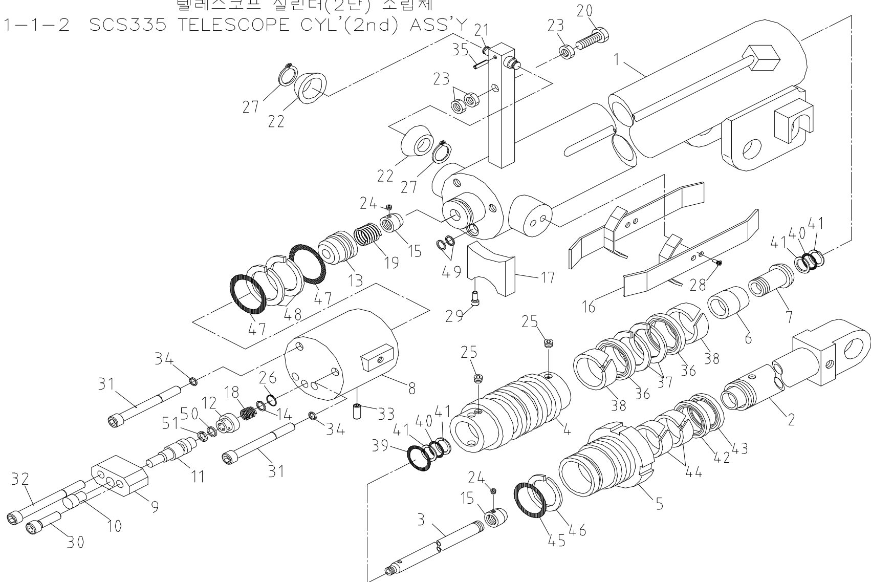
텔레스코프 실린더(2단) 조립체
