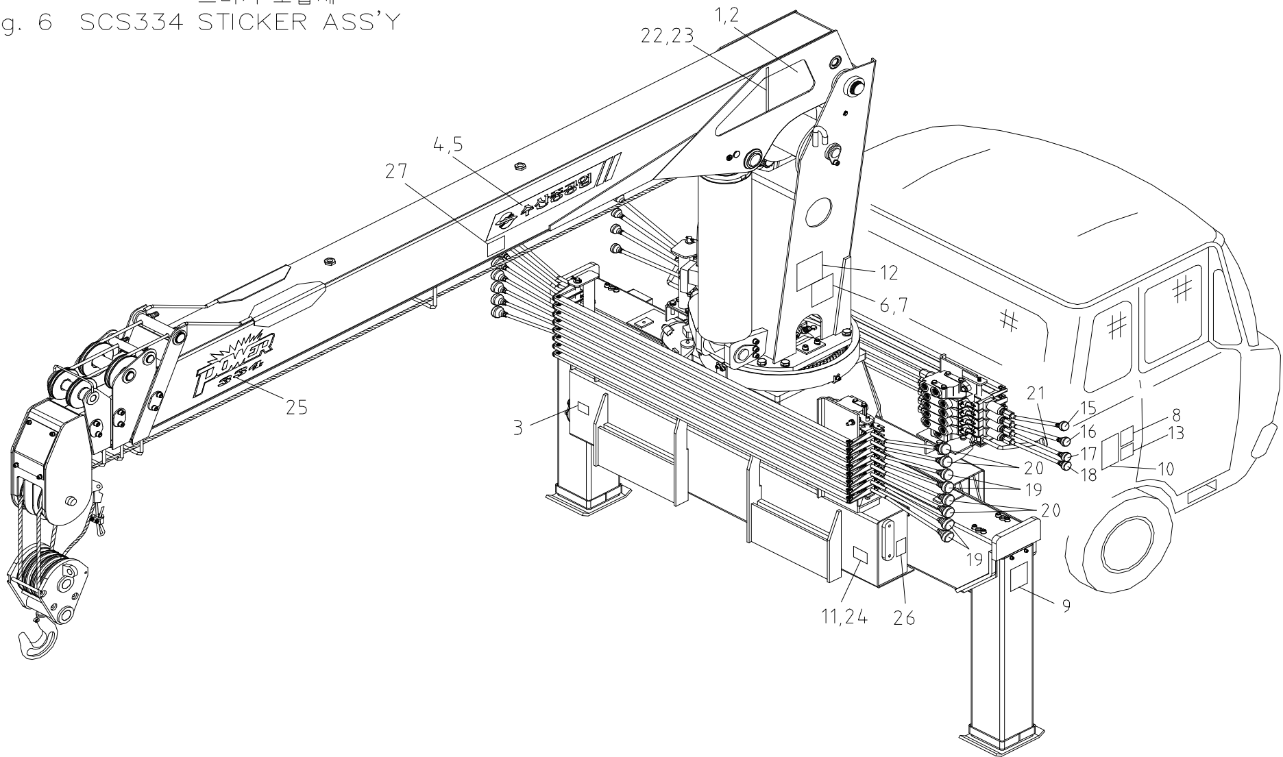
스티커 조립체
