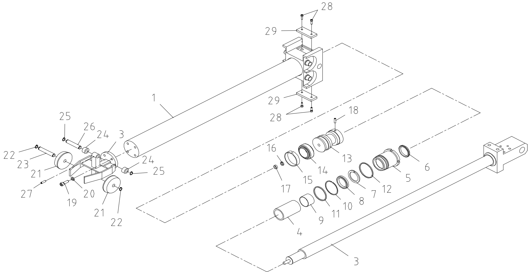
텔레실린더 조립체 Fig. 1-1 SCS333 TELE' CYL' ASS'Y
