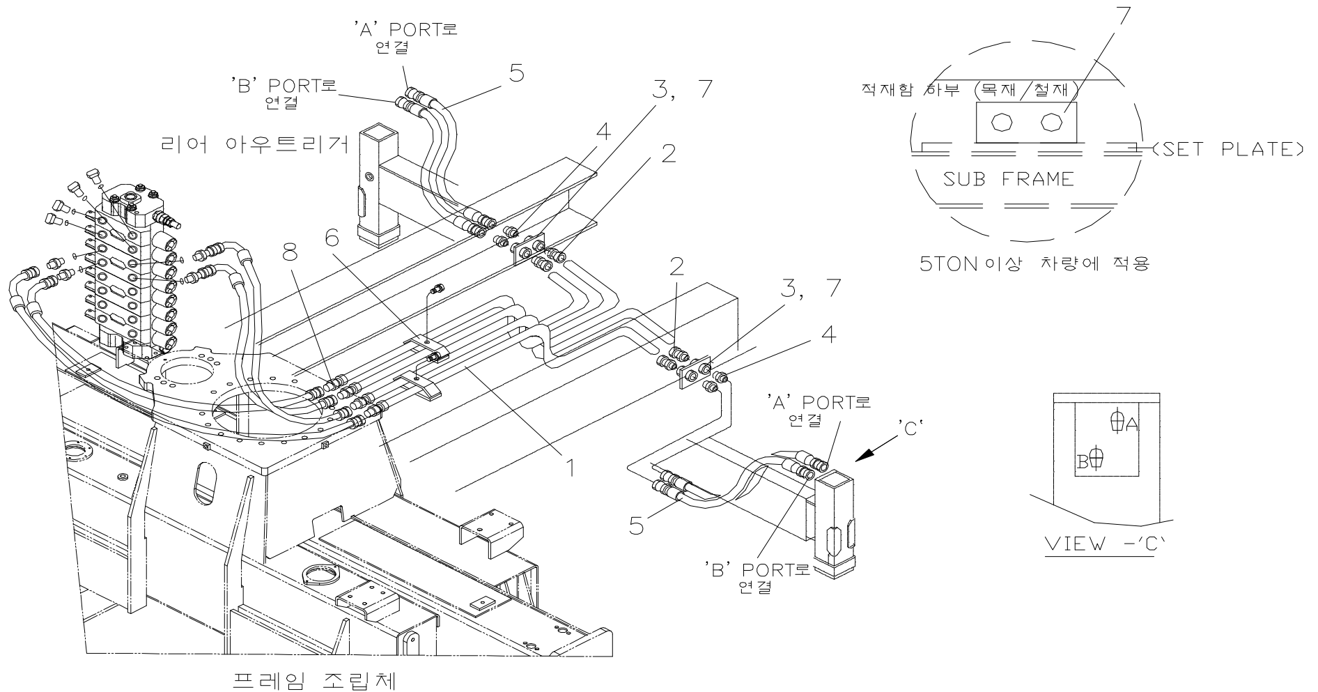
후방 장착 배관 파트 Fig. 8-4 SCS333 R/O M/T PIPING PART
