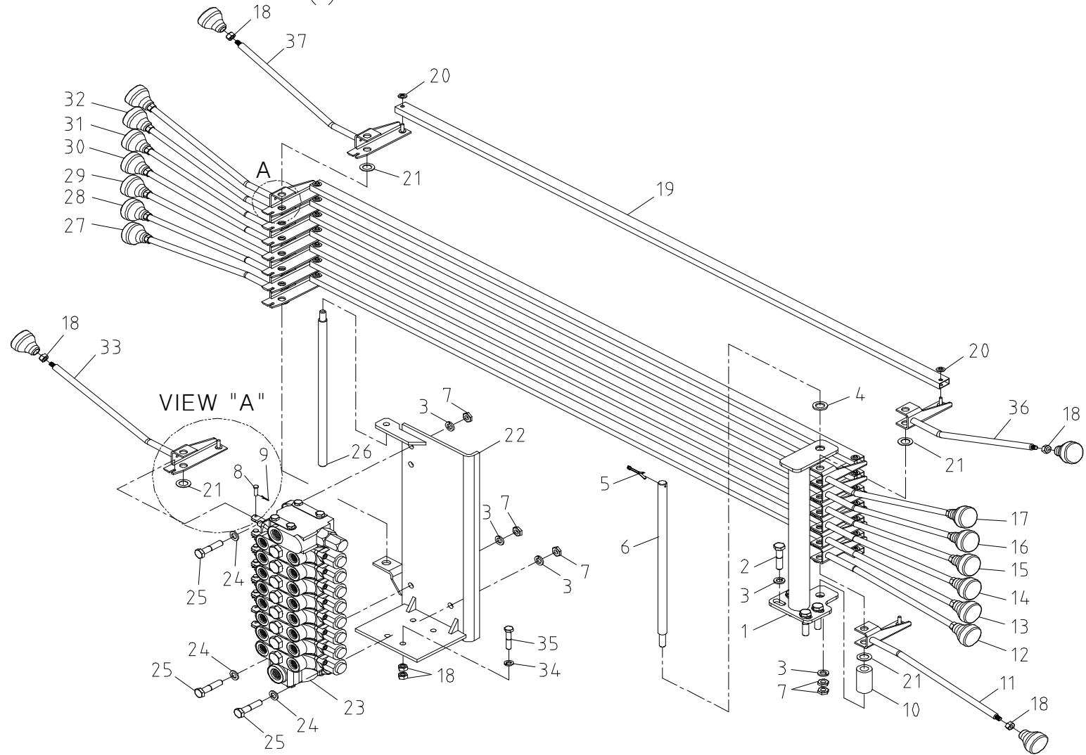
오퍼레이션 조립체(I) Fig. 3-4 SCS333 OPERATION ASS'Y(I)
