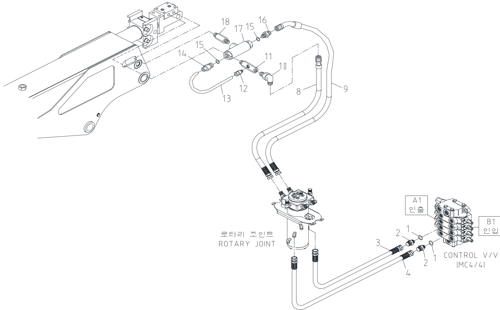
텔레 배관 Fig. 5-4 SCS335 TELE PIPING
