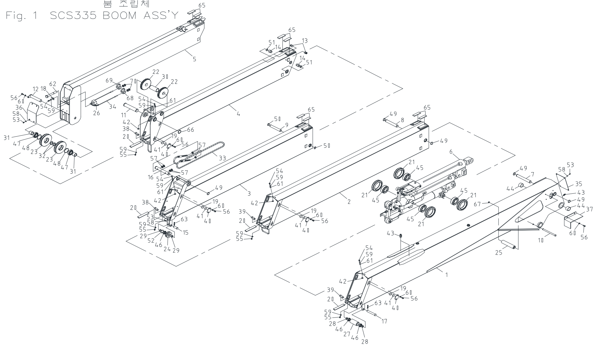
붐 조립체
