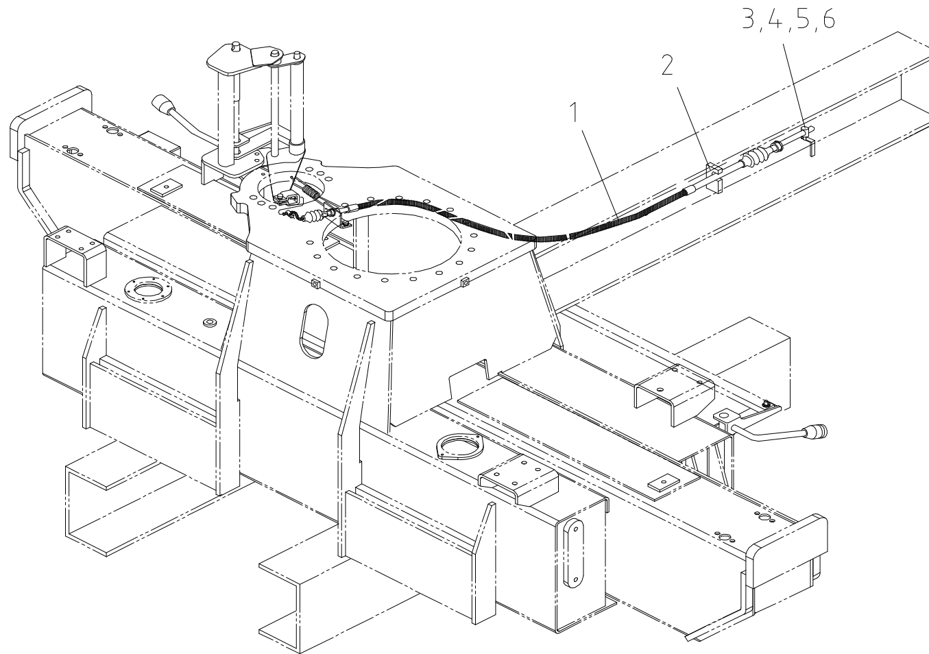
악셀 시스템 파트 Fig. 8-3 SCS333 ACC' SYSTEM PART
