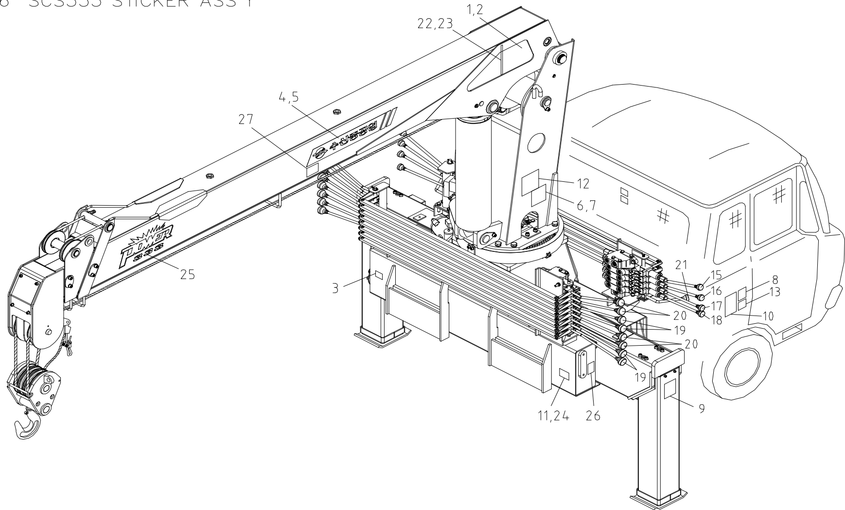
스티커 조립체
