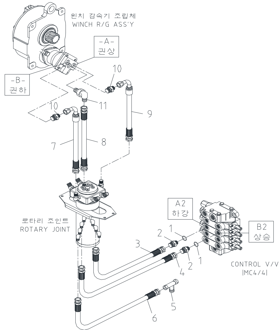
원치 배관 Fig. 5-3 SCS333 WINCH PIPING
