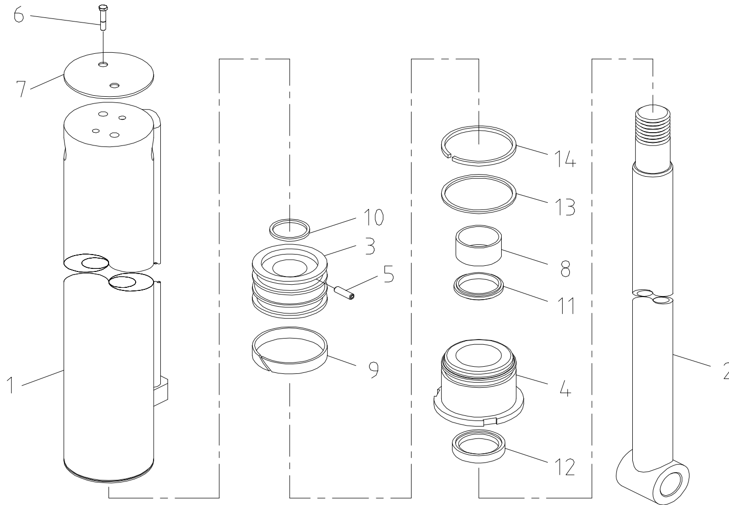
잭 실린더 조립체 Fig. 4-1 SCS333 JACK CYL' ASS'Y
