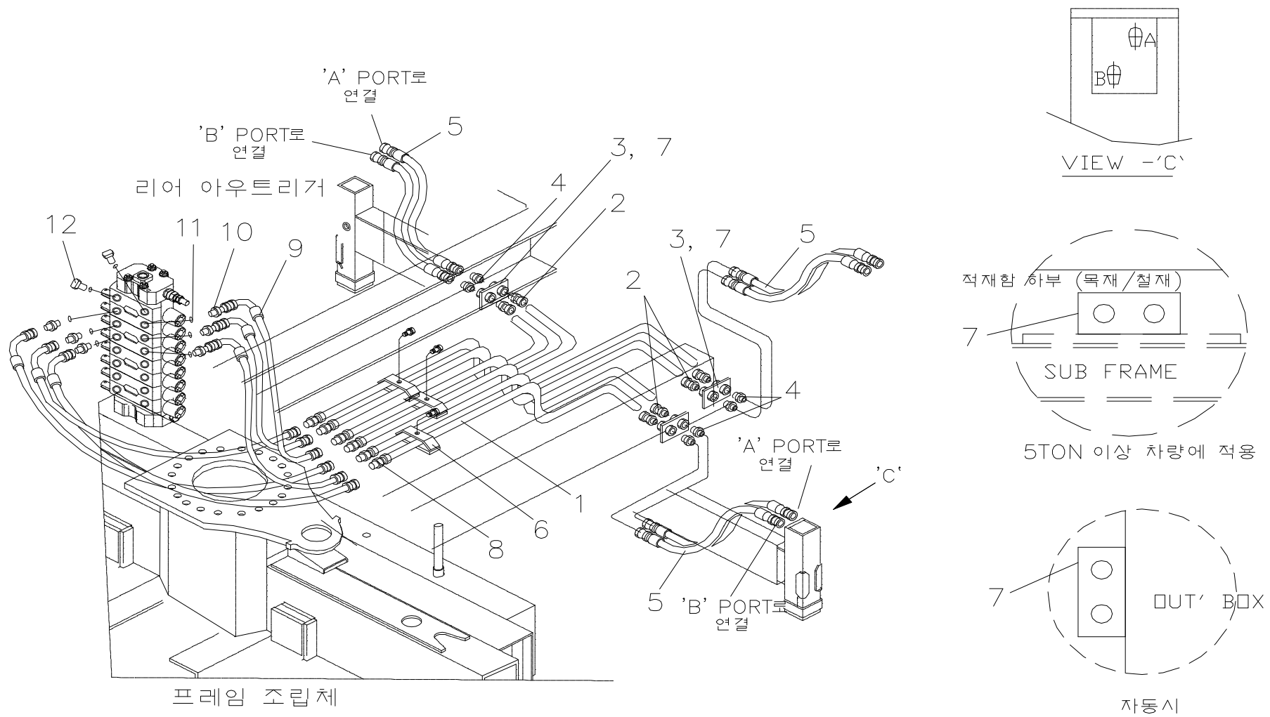
후방 장착 배관 파트 Fig. 8-4 SCS333 R/A M/T PIPING PART
